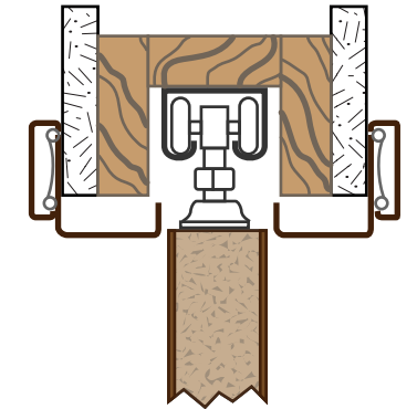
6D Header - Pocket Door Trim
