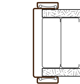
6U Jamb - No Stop
